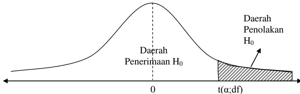
Gambar 2. Daerah Penerimaan dan Penolakan H_0 untuk variabel bebas
