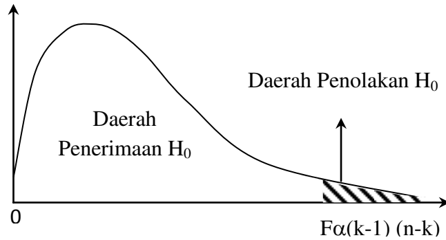
Gambar 1 Daerah Pengujian Penerimaan dan Penolakan H_0 dengan Uji F
