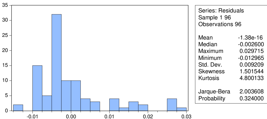
Gambar 5. Hasil Uji Normalitas
