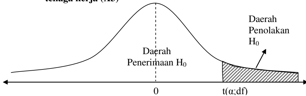
Gambar 4. Daerah Penerimaan dan Penolakan H_0 untuk Variabel jumlah tenaga kerja (X3)
