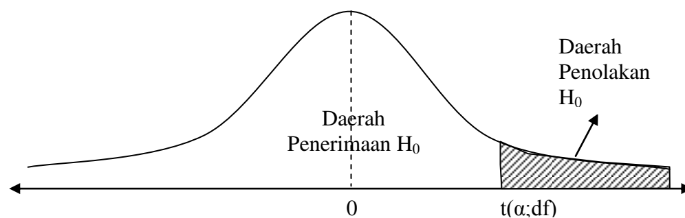
Gambar 3. Daerah Penerimaan dan Penolakan H_0 untuk Variabel lama usaha( X_2 )
