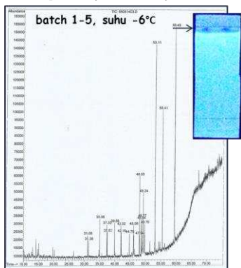
Gambar 1. Hasil analisa GC-MS fraksi squalene
