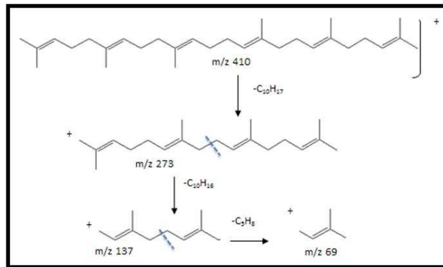
Gambar 3 Mekanisme fragmentasi Squalene
