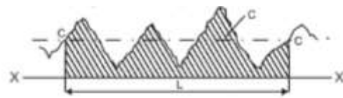
Gambar 2.4 Profil kekasaran permukaan rata-rata Ra (Handoko, Prayoga, 2008)
