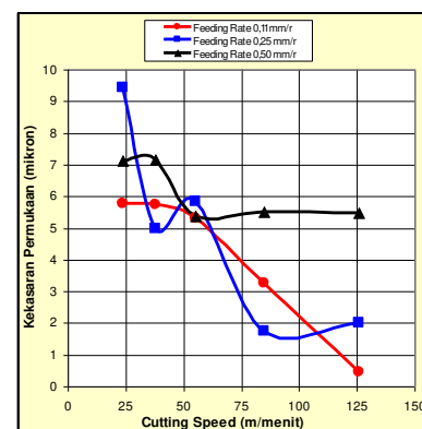
Gambar 4.1 Grafik cutting speed terhadap kekasaran permukaan
