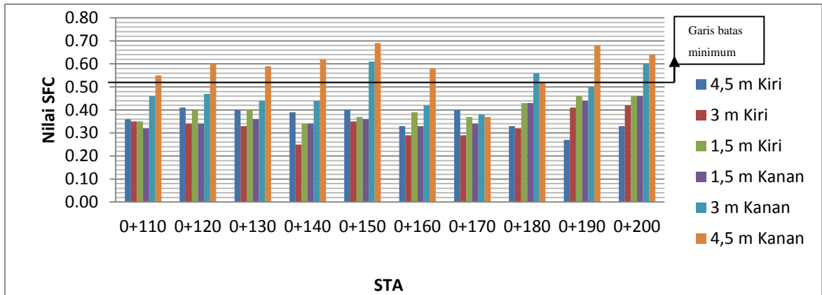
Gambar 1 Grafik nilai SFC sesudah pembersihan rubber deposit pada STA 0 + 110 – STA 0 + 200 Bandar Udara Sultan Syarif Kasim II, Pekanbaru (Persentase lokasi yang bermasalah adalah sebesar 92%)
