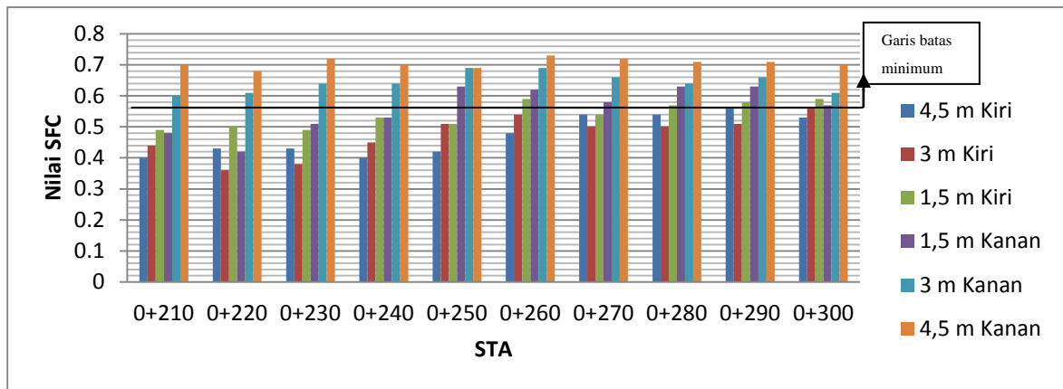
Gambar 2 Grafik nilai SFC sesudah pembersihan rubber deposit pada STA 0 + 210 – STA 0 + 300 Bandar Udara Sultan Syarif Kasim II, Pekanbaru (Persentase lokasi yang bermasalah adalah sebesar 50%)
