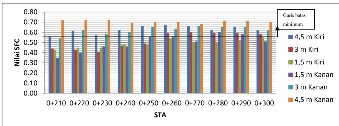
Gambar 6 Grafik nilai SFC sebelum pembersihan rubber deposit pada STA 0 + 210 – STA 0 + 300 Bandar Udara Sultan Syarif Kasim II, Pekanbaru (Persentase lokasi yang bermasalah adalah sebesar 38%)
