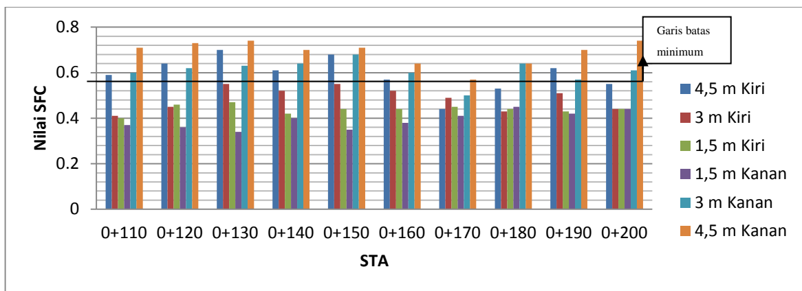
Gambar 5 Grafik nilai SFC sebelum pembersihan rubber deposit pada STA 0 + 110 – STA 0 + 200 Bandar Udara Sultan Syarif Kasim II, Pekanbaru (Persentase lokasi yang bermasalah adalah sebesar 57%)
