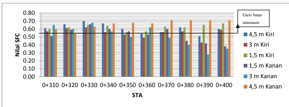
Gambar 3 Grafik nilai SFC sesudah pembersihan rubber deposit pada STA 0 + 310 – STA 0 + 400 Bandar Udara Sultan Syarif Kasim II, Pekanbaru (Persentase lokasi yang bermasalah adalah sebesar 32%)
