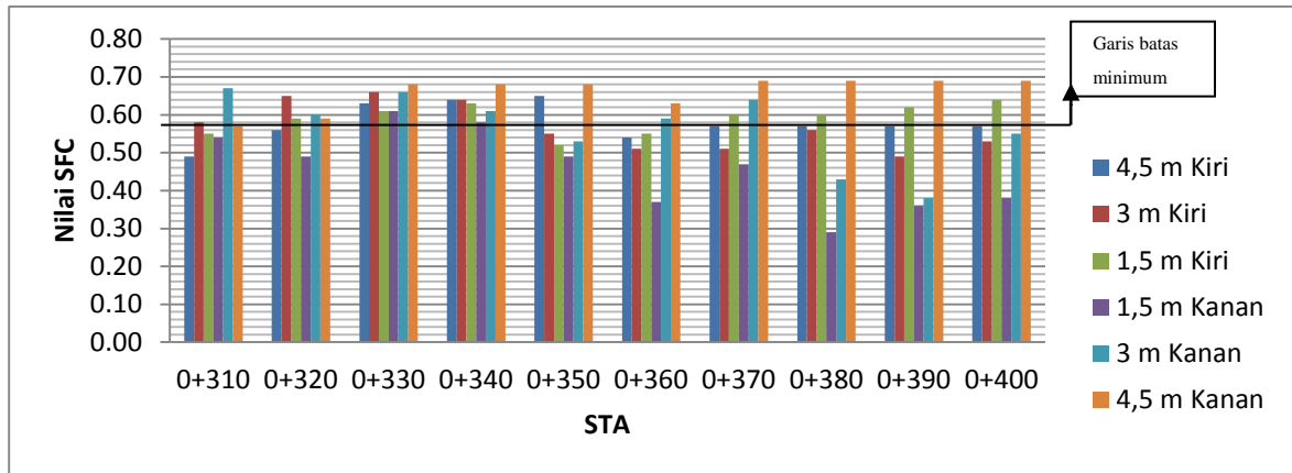
Gambar 7 Grafik nilai SFC sebelum pembersihan rubber deposit pada STA 0 + 310 – STA 0 + 400 Bandar Udara Sultan Syarif Kasim II, Pekanbaru (Persentase lokasi yang bermasalah adalah sebesar 38%)
