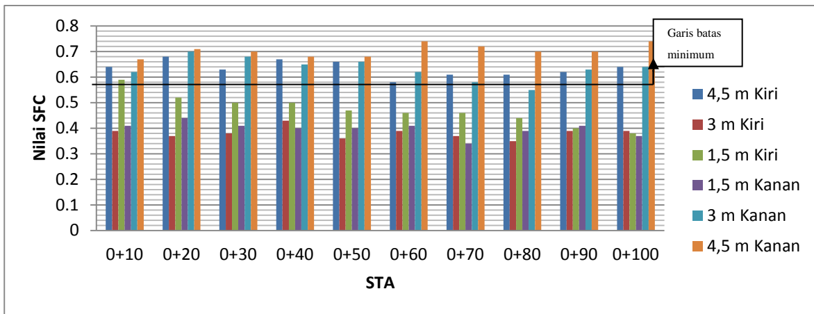
Gambar 4 Grafik nilai SFC sebelum pembersihan rubber deposit pada STA 0 + 10 – STA 0 + 100 Bandar Udara Sultan Syarif Kasim II, Pekanbaru (Persentase lokasi yang bermasalah adalah sebesar 50%)
