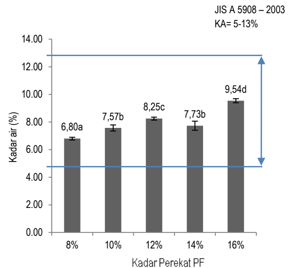
Gambar 2. Grafik kadar air papan partikel. Keterangan. a, b, c, d. Notasi yang sama menunjukkan pengaruh tidak berbeda nyata antar perlakuan berdasarkan uji DMRT taraf kepercayaan 5%.
