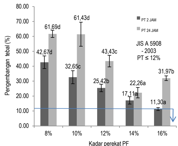
Gambar 4. Grafik rata-rata pengembangan tebal papan partikel. Keterangan. a, b, c, d. Notasi yang sama menunjukkan pengaruh tidak berbeda nyata antar perlakuan berdasarkan uji DMRT taraf kepercayaan 5%.
