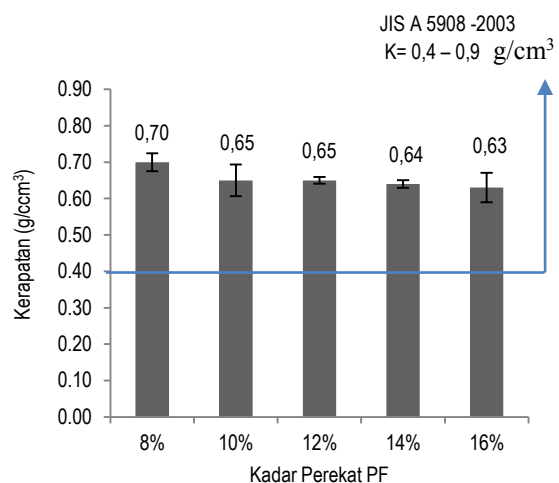
Gambar 1. Grafik rata-rata kerapatan papan partikel.
