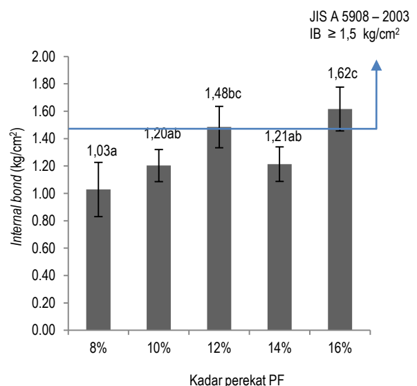
Gambar 7. Grafik rata-rata internal bond (IB) papan partikel.
