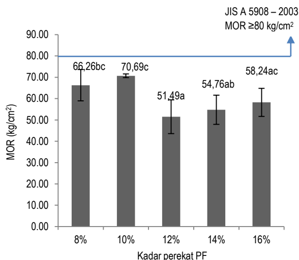
Gambar 6. Grafik rata-rata MOR papan partikel
