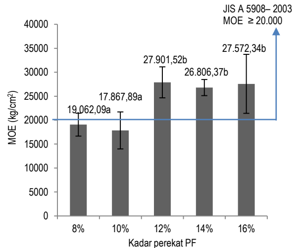
Gambar 5. Grafik rata-rata modulus lentur (MOE) papan Partikel. Keterangan. a, b. Notasi yang sama menunjukkan pengaruh tidak berbeda nyata antar perlakuan berdasarkan uji DMRT taraf kepercayaan 5%.
