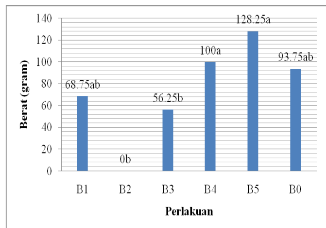
Gambar 5. Grafik rata-rata berat panen jamur tiram putih pada berbagai perlakuan.
