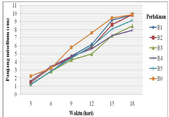
Gambar. 2. Grafik pengamatan pertumbuhan miselium jamur tiram putih ( Pleurotus ostreatus ) pada kultur F2.
