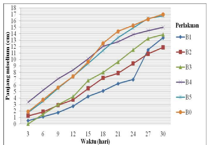
Gambar. 3. Grafik pengamatan pertumbuhan miselium jamur tiram putih ( Pleurotus ostreatus ) pada kultur F3.
