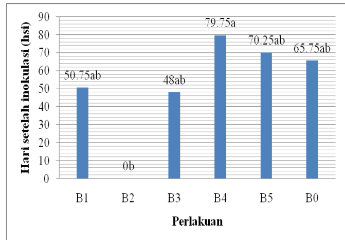
Gambar 4. Grafik rata-rata umur panen jamur tiram putih pada berbagai perlakuan.
