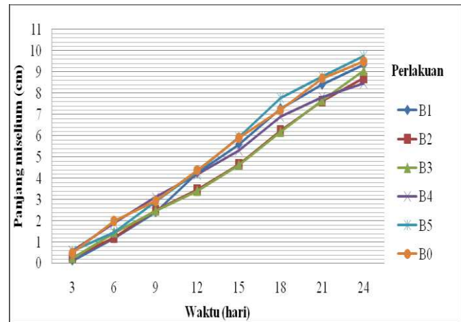
Gambar. 1. Grafik pengamatan pertumbuhan miselium jamur tiram putih ( Pleurotus ostreatus ) pada kultur F1.
