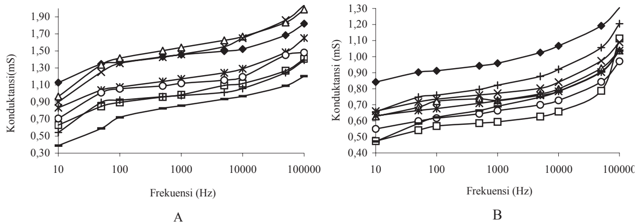
Gambar 2. Spektrum konduktansi listrik dari putih (A) dan kuning (B) telur dengan variasi lama penyimpanan ( \diamond = hari ke-0, \square = hari ke-2, \Delta = hari ke-4, \times = hari ke-6, * = hari ke-8, \circ = hari ke-10, + = hari ke-12, - = hari ke-14) pada frekuensi yang berbeda.
