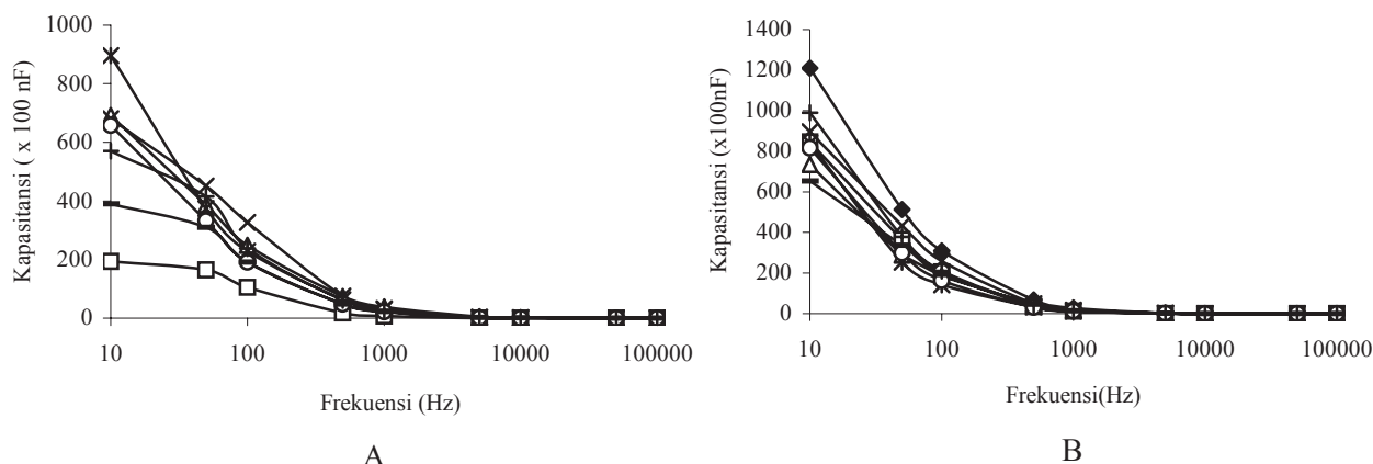
Gambar 3. Spektrum kapasitansi listrik dari putih (A) dan kuning (B) telur dengan variasi lama penyimpanan ( \diamond = hari ke-0, \square = hari ke-2, \Delta = hari ke-4, \times = hari ke-6, * = hari ke-8, \circ = hari ke-10, + = hari ke-12, - = hari ke-14) pada frekuensi yang berbeda.
