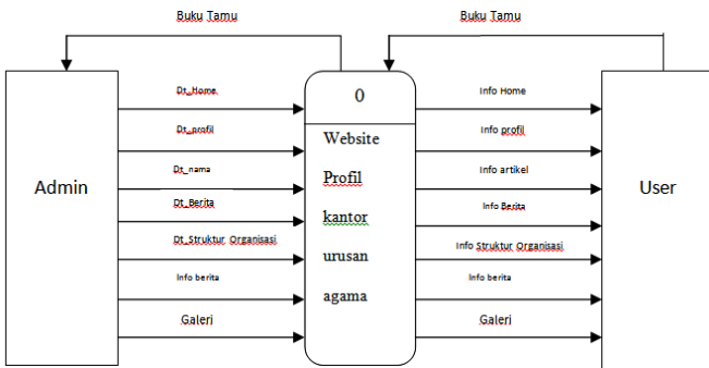
Gambar 1 Diagram Konteks
