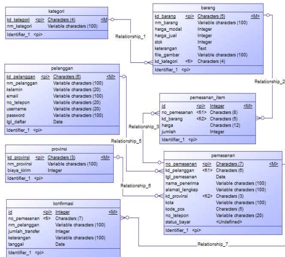
Gambar 7. Diagram ERD Sumber : Diolah, 2015
