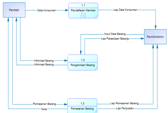
Gambar 5. DFD Level 1 Sumber : Diolah, 2015
