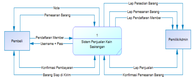
Gambar 4. Diagram Kontek Model E-Commerce UKM Produk Sasirangan Sumber : Diolah, 2015
