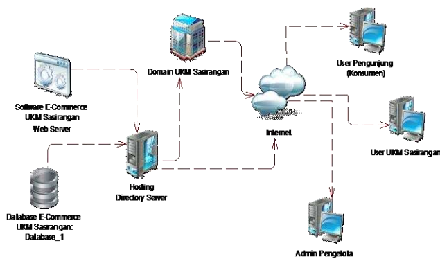
Gambar 3. Arsitektur Model E-Commerce UKM Produk Sasirangan Sumber : Diolah, 2015
