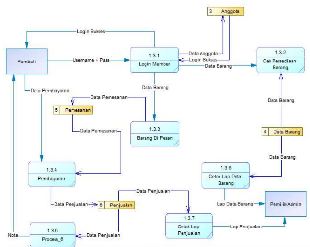
Gambar 6. DFD Level 2 Sumber : Diolah, 2015
