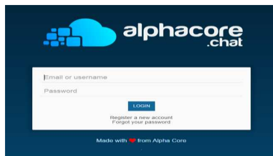
Gambar 3. Halaman Login
