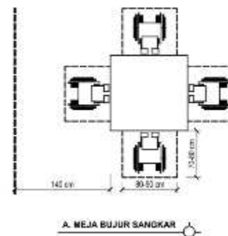
Gambar 4. Standart meja persegi untuk kelas SLB
