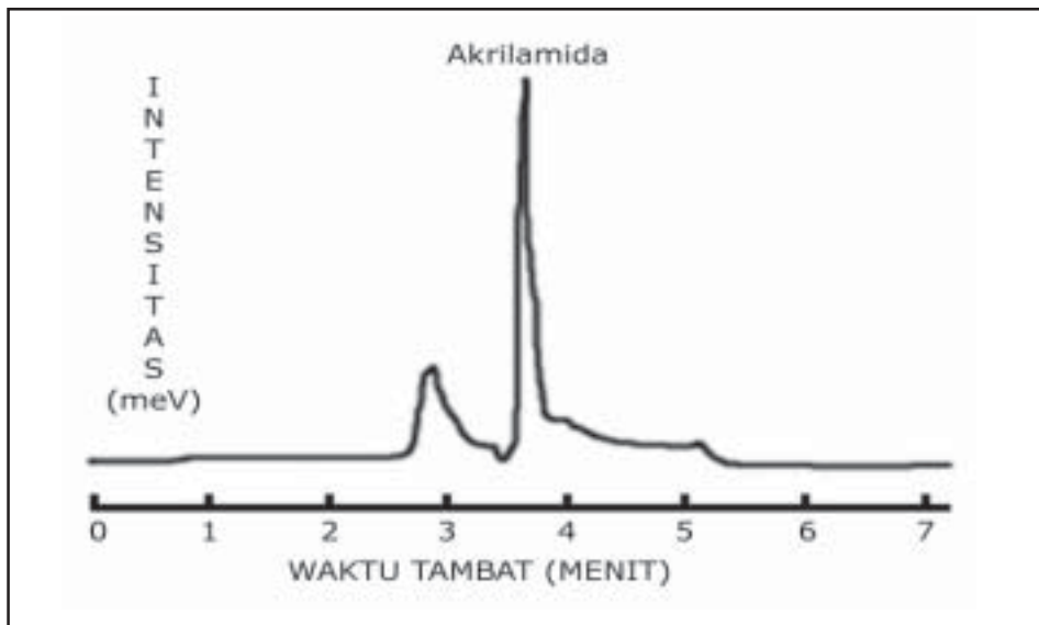
Gambar 1. Kromatogram akrilamida 6 ppm dengan fase gerak asetonitril-air-asam fosfat (5:94:1), pelarut asam fosfat 10%, volume penyuntikkan 20 \mu l dan laju alir 1,2 ml/menit
