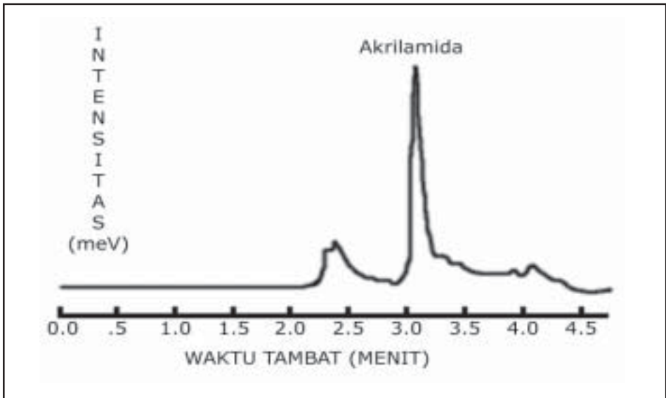
Gambar 3. Kromatogram akrilamida yang ditambahkan ke dalam keripik kentang blanko dengan fase gerak asetronitril-air-asam fosfat (5:94:1), pelarut asam fosfat 10%, volume penyuntikan 20 \mu l dan laju alir 1,2 ml/menit
