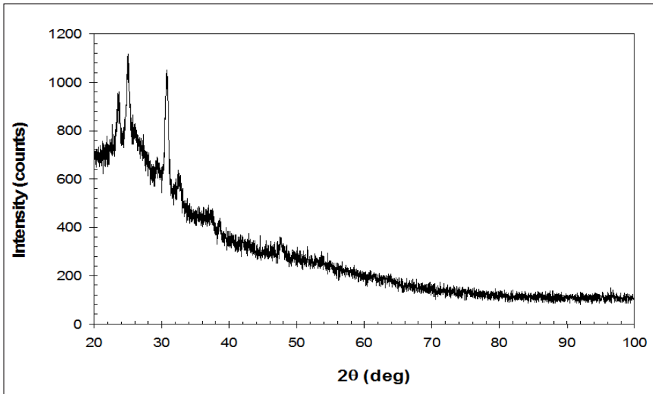
Gambar 3. Pola difraktogram nanosuspensi kering asam mefenamat-PVP 1% dengan waktu sonikasi 1 jam
