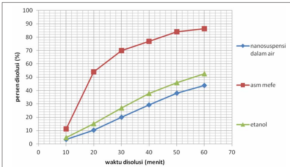
Gambar 4. Kurva profil disolusi dari bahan baku asam mefenamat, nanosuspensi kering asam mefenamat dalam pelarut organik dan sampel nanosuspensi kering asam mefenamat
