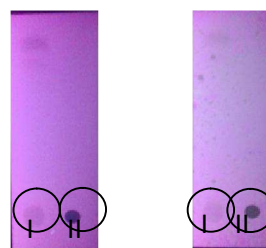
(a) (b) Gambar 3. Hasil KLT deteksi flavonoid fase diam selulosa, fase gerak asam asetat 15%, pembandingan rutin, deteksi di bawah UV 366 nm dan disemprot sitroborat diambil di bawah UV 366 I. Ekstrak etanol daun sirih merah II. Rutin (a) Deteksi di bawah lampu sinar UV 366 nm (b) Setelah disemprot dengan pereaksi sitroborat pada sinar UV 366 nm
