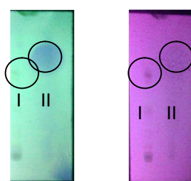
Gambar 4. (a) Hasil KLT deteksi senyawa minyak atsiri dengan fase diam silika gel F 254 , fase gerak toluen-etil asetat, pembanding eugenol diamati dibawah UV 254 dan
