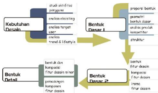
Gambar 4. Metodologi perancangan
