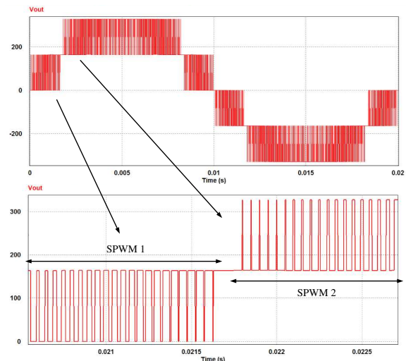
Gambar 6. Keluaran full bridge inverter lima tingkat
