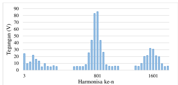
Gambar 8. Spektrum harmonisa tegangan
