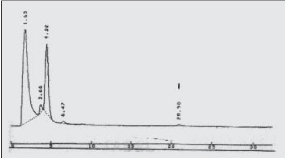
Gambar 7 : Kromatogram kafeina (I) pada sampel E. Volume penyuntikan : 20 \mu l. kondisi : kolom Latek C18 (15 cm x 4,0 mm), fase gerak campuran asetonitril dan dapar asetat pH 5 (5:95), kecepatan aliran 1 ml/menit, detector spektrofotometer UV 254 nm, dengan sensitivitas 0,04.
