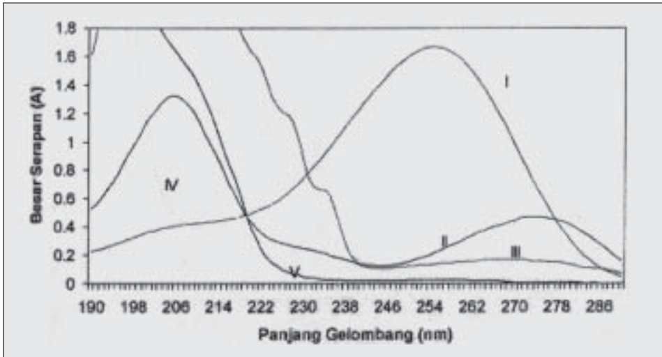
Gambar 1 : Kurva serapan larutan asam sorbet 10,05 ppm (I), kofeina 10,01 ppm (II), sakarin 9,64 ppm (III), asam benzoat 10,01 ppm (IV), dan aspartame 10,03 ppm (V) dalam pelarut aquabides pada panjang gelombang 190-290 nm.
