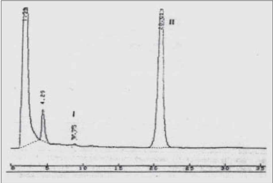
Gambar 5 : Kromatogram asam benzoat (I) dan kofeina (II) pada sampel C. Volume penyuntikan : 20 \mu l. kondisi : kolom Latek C18 (15 cm x 4,0 mm), fase gerak campuran asetonitril dan dapar asetat pH 5 (5:95), kecepatan aliran 1 ml/menit, detector spektrofotometer UV 254 nm, dengan sensitivitas 0,04.
