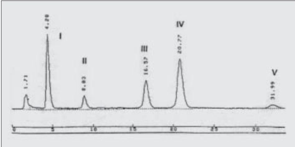
Gambar 2 : Kromatogram campuran standar sakarin 27,35 ppm (I), asam benzoate 15,21 ppm (II), asam sorbat 1,02 ppm (III), kofeina 10,1 ppm (IV), aspartame 50,4 ppm (V). Volume penyuntikan : 20 \mu l. kondisi : kolom Latek C18 (15 cm x 4,0 mm), fase gerak campuran asetonitril dan dapar asetat pH 5 (5:95), kecepatan aliran 1 ml/menit, detector spektrofotometer UV 254 nm, dengan sensitivitas 0,04.
