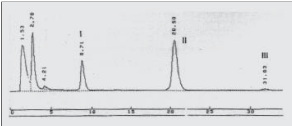
Gambar 6 : Kromatogram asam benzoate (I), kofeina (II) dan aspartame (III) pada sampel D. Volume penyuntikan : 20 \mu l. kondisi : kolom Latek C18 (15 cm x 4,0 mm), fase gerak campuran asetonitril dan dapar asetat pH 5 (5:95), kecepatan aliran 1 ml/menit, detector spektrofotometer UV 254 nm, dengan sensitivitas 0,04.
