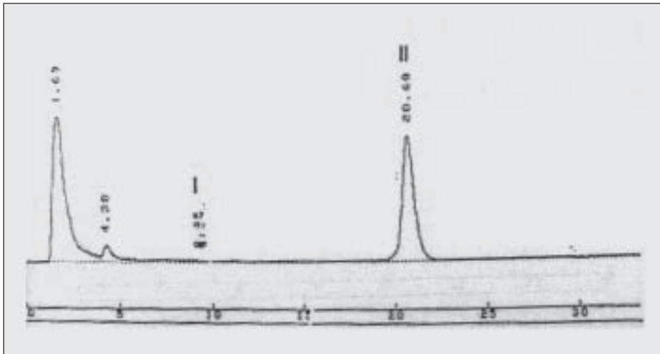
Gambar 3 : Kromatogram asam benzoat (I) dan kafeina (II) pada sampel A. Volume penyuntikan : 20 \mu l. kondisi : kolom Latek C18 (15 cm x 4,0 mm), fase gerak campuran asetonitril dan dapar asetat pH 5 (5:95), kecepatan aliran 1 ml/menit, detector spektrofotometer UV 254 nm, dengan sensitivitas 0,04.
