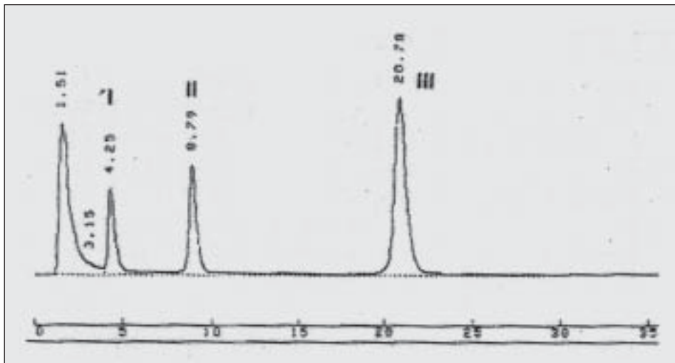
Gambar 4 : Kromatogram sakarin (I), asam benzoate (II) dan kafeina (III) pada sampel B. Volume penyuntikan : 20 \mu l. kondisi : kolom Latek C18 (15 cm x 4,0 mm), fase gerak campuran asetonitril dan dapar asetat pH 5 (5:95), kecepatan aliran 1 ml/menit, detector spektrofotometer UV 254 nm, dengan sensitivitas 0,04.
