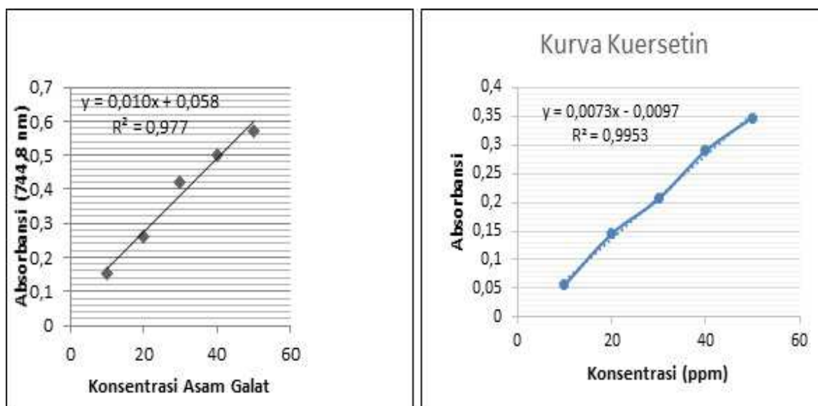
Gambar 1. Kurva kalibrasi asam galat pada panjang gelombang 744,8 nm dan kuersetin galat pada panjang gelombang 431 nm
