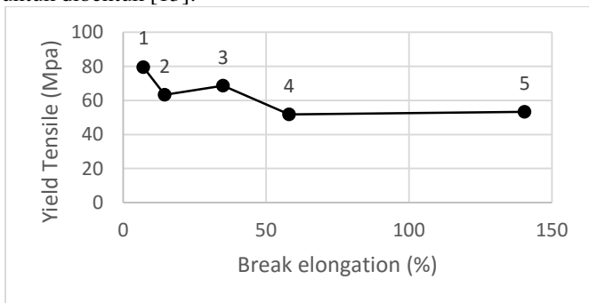
Gambar 4 Hasil Uji Tarik
