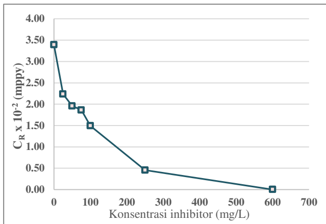
Gambar 4. Grafik hubungan variasi konsentrasi inhibitor ekstrak kulit dalam semangka dengan laju korosi dalam 2% NaCl dari metode polarisasi potensiodinamik.
