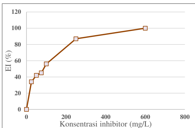
Gambar 5. Grafik hubungan variasi konsentrasi inhibitor ekstrak kulit dalam semangka dengan laju reaksi dalam 2% NaCl dari metode polarisasi potensiodinamik
