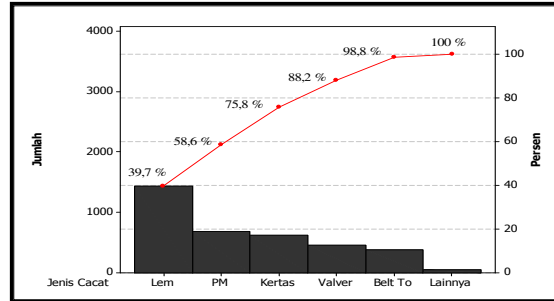
Gambar 6b. Diagram Pareto tahap 2
