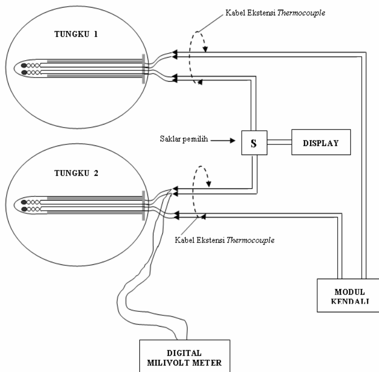
Gambar 2. Pengukuran emf pada Keluaran Thermocouple Tungku 2
