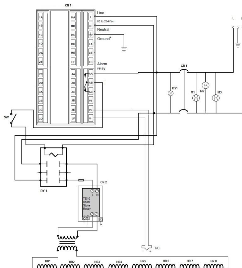
Gambar wiring sistem tungku thermolyne secara lengkap ditunjukkan gambar 3 dibawah ini.
