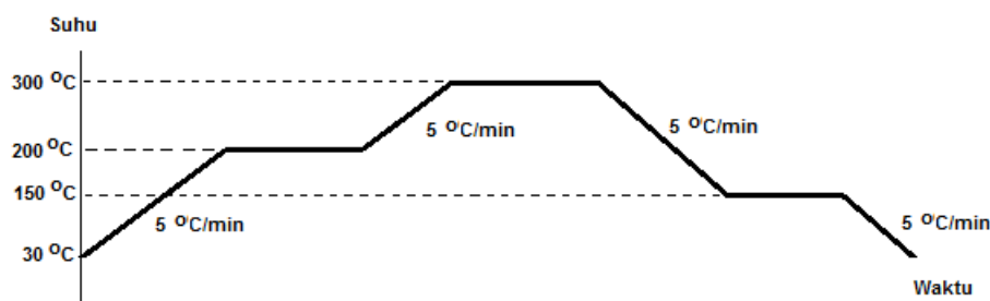
Gambar.4. Pola kerja modul kendali Tungku Thermolyne [3]
