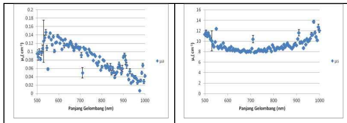
Gambar. 4 Absorbtion dan scattering coefficient untuk kelima pengukuran pada phantom-1 dengan kondisi kedua.
