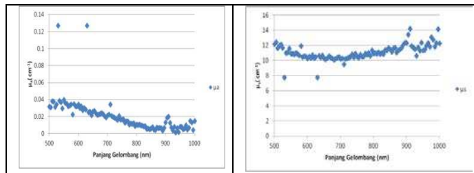
Gambar. 8. Absorbtion dan scattering coefficient hasil ekstraksi phantom-3.
