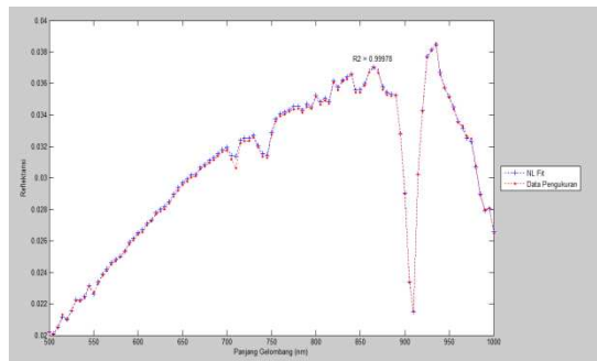
Gambar. 3. Fitting pada kondisi keempat dengan jarak 1 cm.
