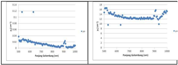
Gambar. 6. Absorbtion dan scattering coefficient hasil ekstraksi phantom-2.
