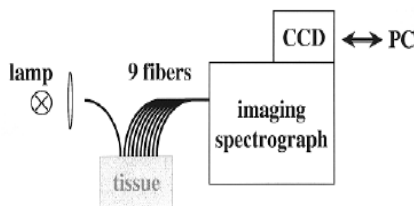
Gambar. 2. Konfigurasi pengukuran DOS pada Doornbos [12].
