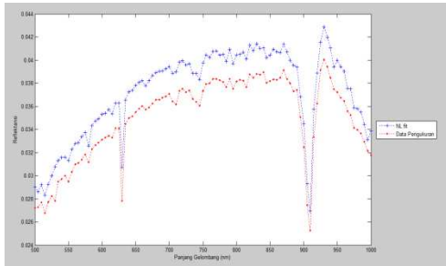
Gambar. 7. Proses fitting pada phantom-3 dengan jarak 1 cm.
