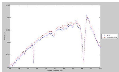
Gambar. 5. Proses fitting pada phantom-2 jarak 1 cm.
