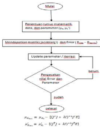
Gambar. 1. Flowchart algoritma Lavenberg Marquardt secara umum.
