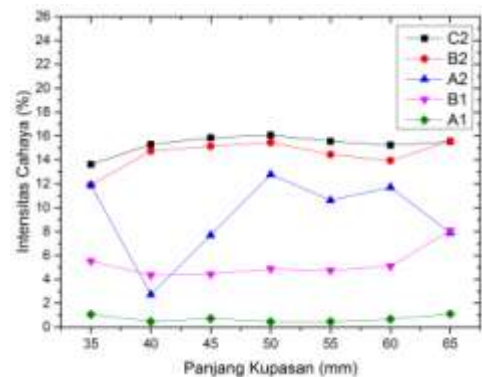
Gambar 8. Grafik Pengaruh Panjang Kupasan terhadap Prosentase Intensitas Cahaya Pada Tiap Output dengan Port C1 sebagai Sinyal Input
