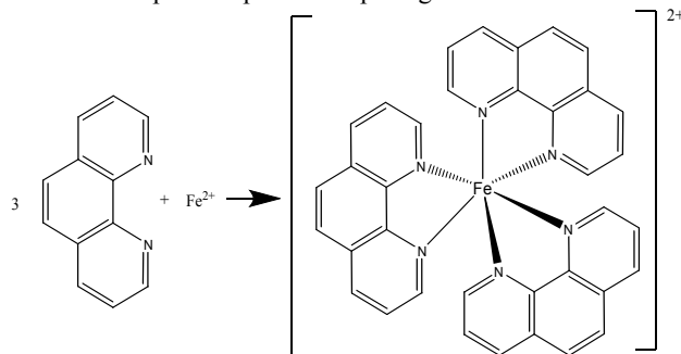
Gambar 3 Reaksi Pembentukan Kompleks [\text{Fe}(\text{fenantrolin})_3]^{2+}
