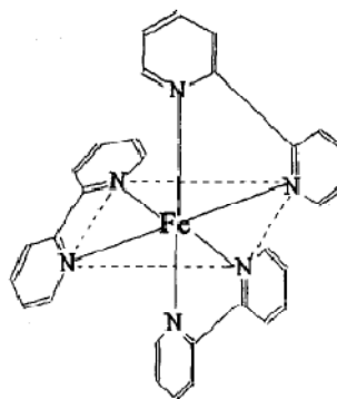
Gambar 4 Bentuk Geometri Molekul [\text{Fe}(\text{fenantrolin})_3]^{2+}
