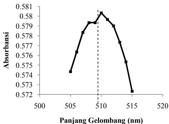
Gambar 2 Kurva Penentuan Panjang Gelombang Maksimum Kompleks [\text{Fe}(\text{fenantrolin})_3]^{2+} pada Rentang Panjang Gelombang 505-515 nm dengan interval 1 nm
