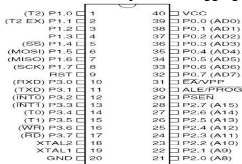
Gambar 1. Mikrokontroler Atmel AT89S8252
