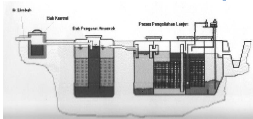
Gambar 2 : Diagram Proses Pengolahan Air Limbah Rumah Sakit.
