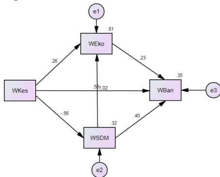
Gambar . 7. Model Spasial pada Persamaan Struktural
