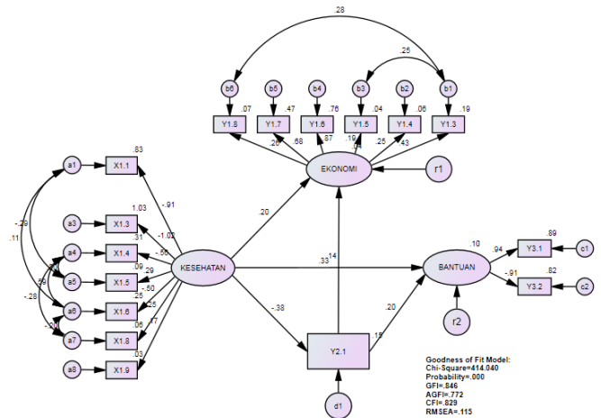
Gambar. 6. Model Struktural Hasil Modifikasi dan Signifikan
