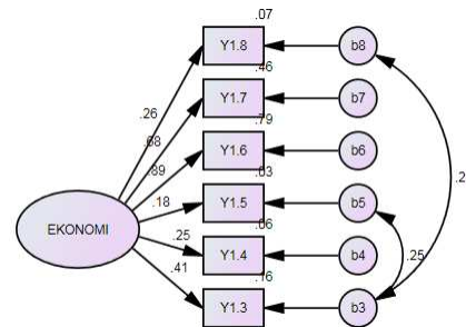
Gambar. 4. Model CFA Variabel Laten Ekonomi Setelah Modifikasi
