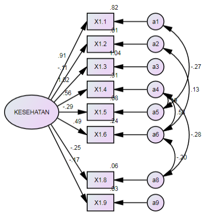
Gambar. 3. Model CFA Variabel Laten Kesehatan Setelah Modifikasi
