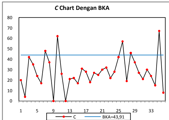
Gambar 5. Diagram Kontrol c Dengan BKA
