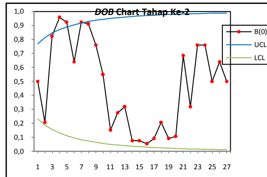
Gambar 4. Diagram DOB Pada Tahap Ke-2
