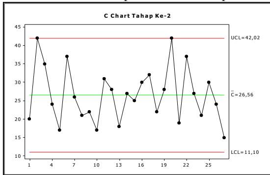
Gambar 3.Diagram Kontrol c Univariat Tahap Ke-2
