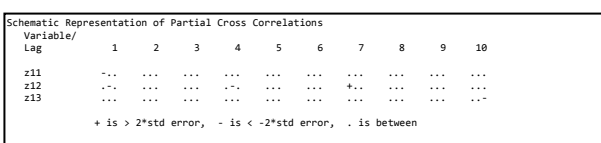
Gambar 4. Plot MPACF data yang sudah stationer pada VARX pertama
