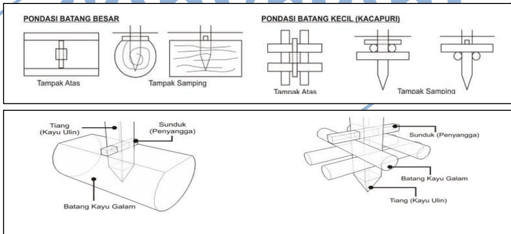
Gb 4. Ilustrasi sistem Pondasi yang diterapkan dalam rumah Bubungan Tinggi (sumber: Faisal Moegis, isalliv8.blogspot.com)
