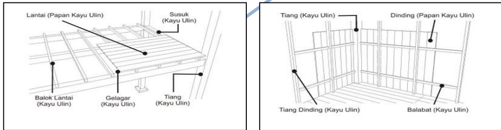
Gb 3. Ilustrasi sistem struktur kayu yang diterapkan dalam rumah Bubungan Tinggi (sumber: Faisal Moegis, isalliv8.blogspot.com)
