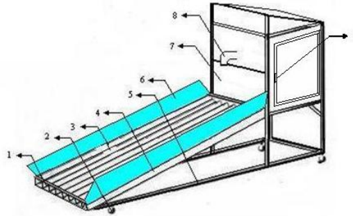
Gambar 2. Pengering dengan kolektor surya
