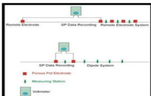
Gambar 5. Amplitudo Potensial (atas) dan Gradien Potensial (bawah)
