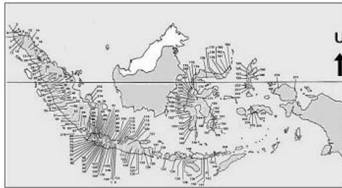
Gambar 3. Penyebaran Panas Bumi di Indonesia (Sumber DESDM)
