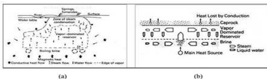
Gambar 2. (a) Model Sistim Dominasi Uap dari White (1971) dan (b) Model Sistim Dominasi D'Amor dan Truesdell (1979 dari Grant et al, 1982)
