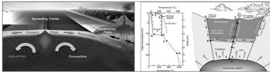
Gambar 1. Proses Pergerakan Lempeng Tektonik (Gambar dari Geothermal Education Office) dan Model Sistim Hidrotermal dari White (1967).
