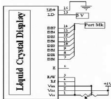
Gambar 3.6 Rangkaian LCD Sumber: Perancangan
