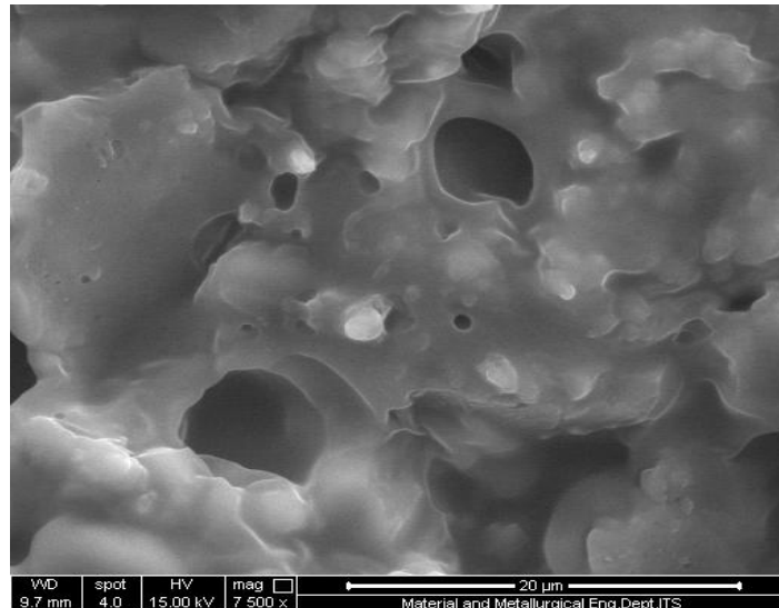
Gambar 1. Hasil SEM 0.7g Biji Kurma dengan matriks PEG pada perbesaran 7500 kali
