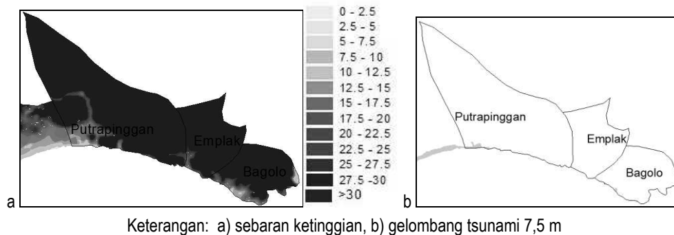
Gambar 9. Perbandingan distribusi genangan gelombang tsunami di desa pantai Kecamatan Kalipucang
