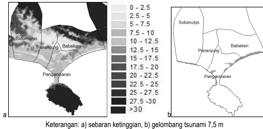
Gambar 8. Perbandingan distribusi genangan gelombang tsunami di desa pantai Kecamatan Pangandaran
