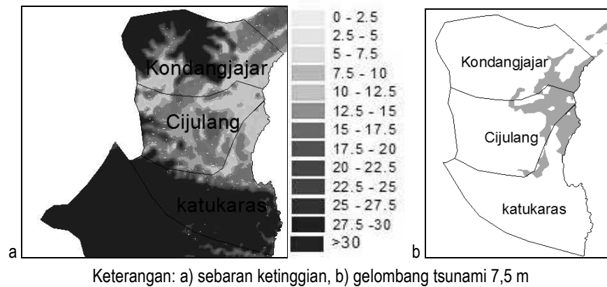
Gambar 5. Perbandingan distribusi genangan gelombang tsunami di desa pantai Kecamatan Cijulang
