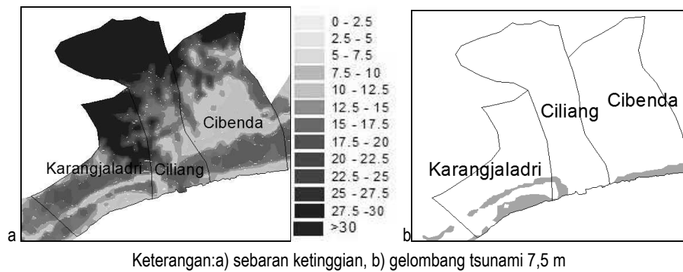
Gambar 6. Perbandingan distribusi genangan gelombang tsunami di desa pantai Kecamatan Parigi
