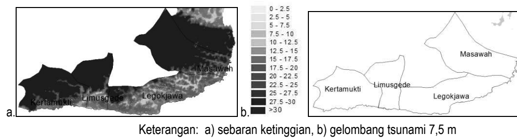
Gambar 4. Perbandingan distribusi genangan gelombang tsunami di desa pantai Kecamatan Cimerak.
