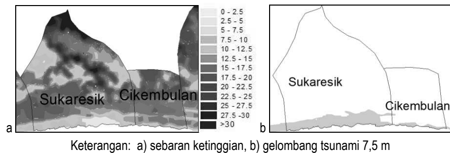
Gambar 7. Perbandingan distribusi genangan gelombang tsunami di desa pantai Kecamatan Parigi
