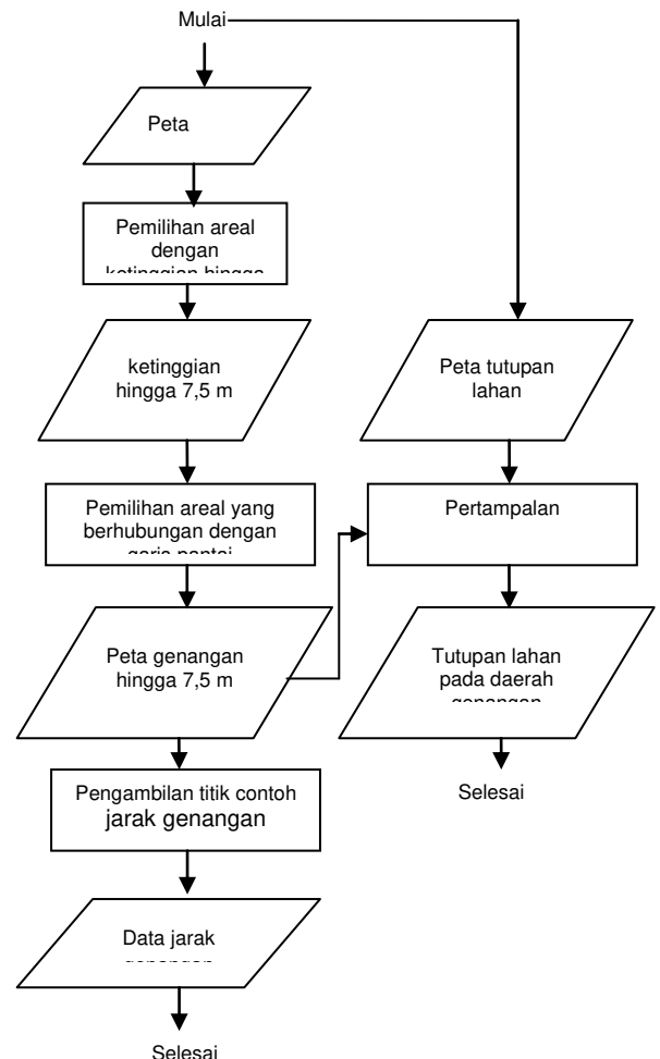
Gambar 1. Metode penentuan potensi kerawanan kerusakan secara spasial
