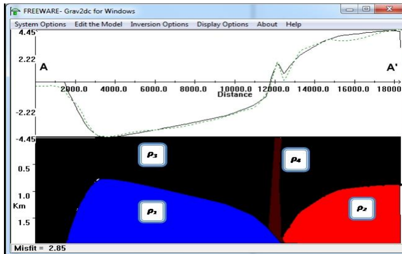
Gambar 7. Pemodelan 2D Penampang A-A'
