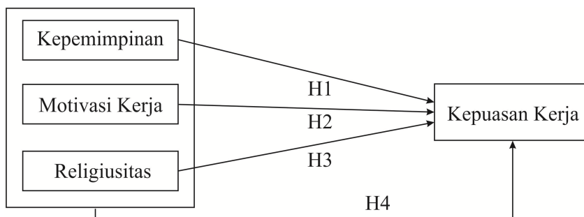
Gambar 2.2. Kerangka Penelitian
