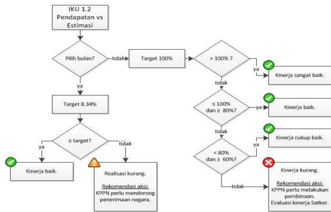
Gambar. 3. Diagram alur analisis IKU 1. 2.
