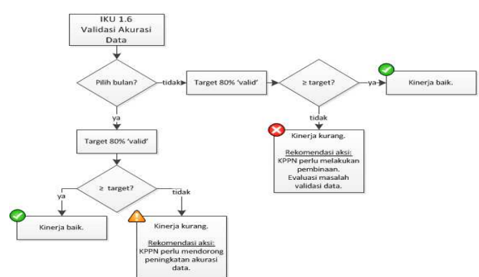
Gambar. 7. Diagram alur analisis IKU 1. 6.
