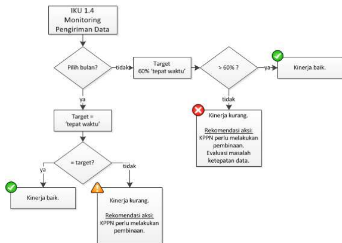
Gambar. 5. Diagram alur analisis IKU 1. 4.
