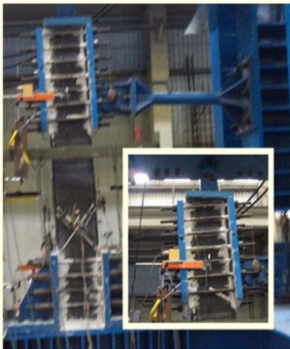
Gambar 5. Kegagalan benda uji C-1C
