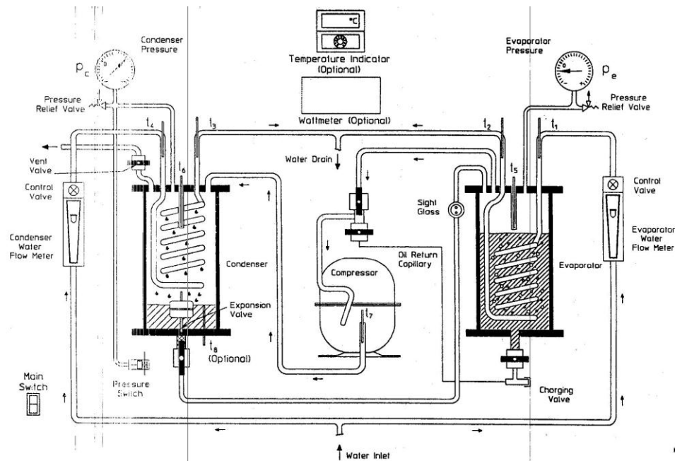
Gambar.2.Mesin Refreigerasi R 633
