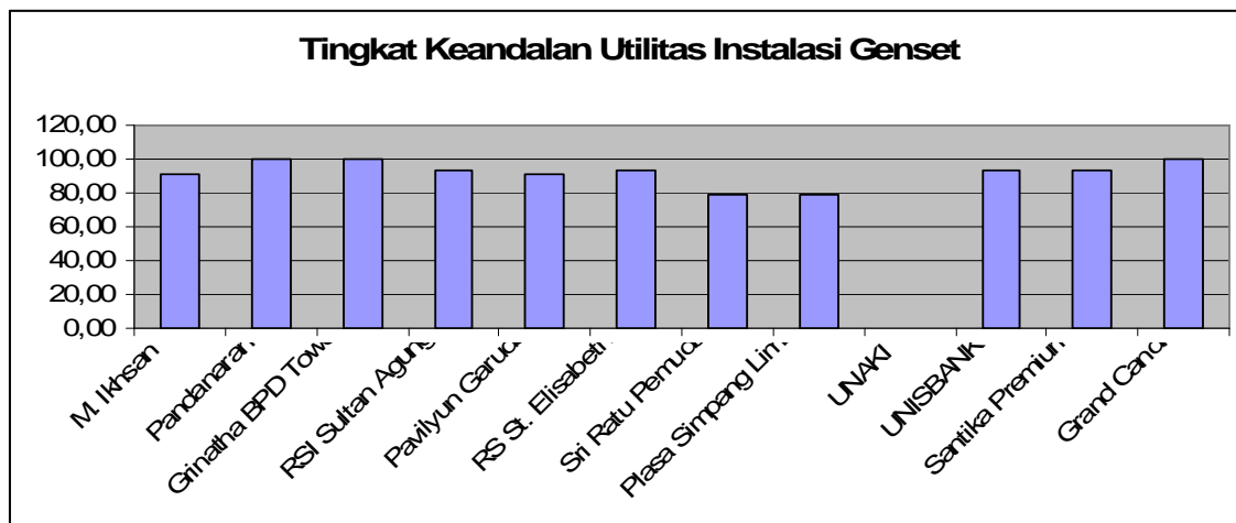
Gambar 2. Tingkat Keandalan Utilitas Instalasi Genset Bangunan Gedung Bertingkat di Kota Semarang
