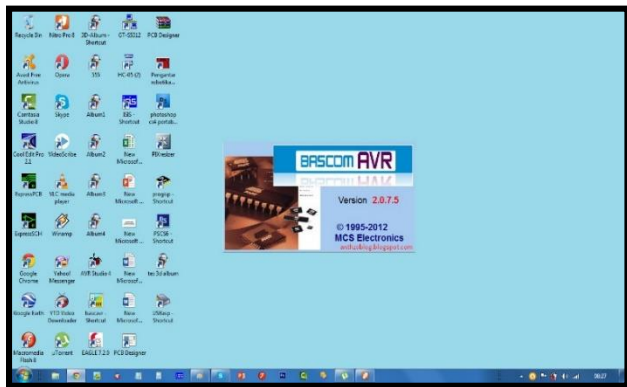
Gambar 8. Menu Utama
