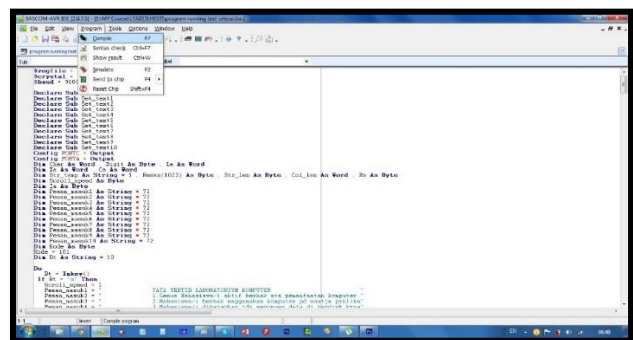
Gambar 12. Mengkompil Program
