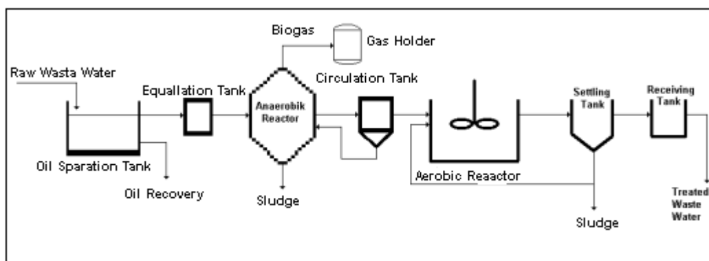
Gambar 2 : Diagram Alir Proses Pengolahan Limbah Cair Industri CPO
