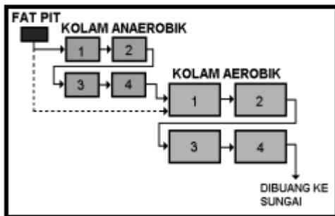
Gambar 1 : Diagram Alir Proses Pengolahan Limbah di PKS PT. Kertajaya 1) .
