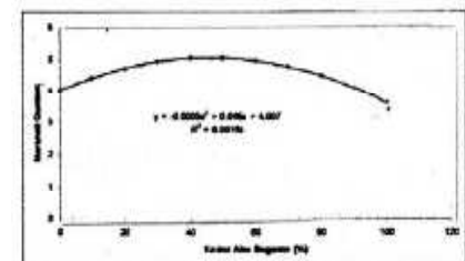
Gambar 5. Hubungan Penambahan Abu Bagasse Dengan Marshall Quotient
