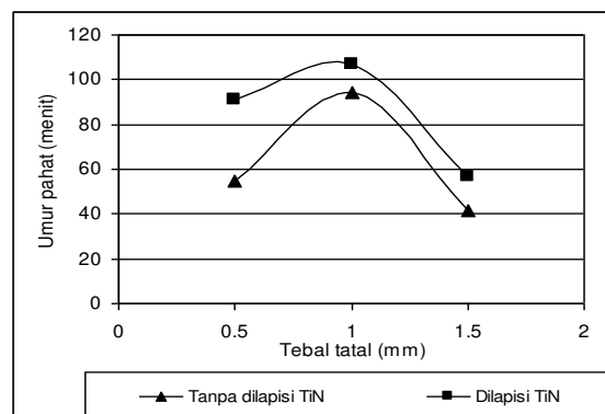
Gambar 6. Grafik tebal tatal vs umur pahat, dilapisi dan tanpa dilapisi kecepatan potong 42 m/min, laju pemakanan 0.090 mm/put
