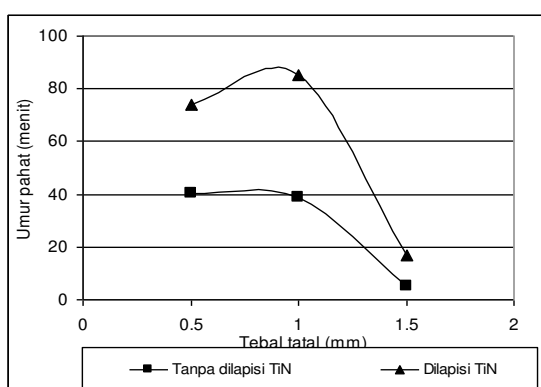
Gambar 5. Grafik tebal tatal vs umur pahat, dilapisi dan tanpa dilapisi kecepatan potong 36 m/min, laju pemakanan 0.090 mm/put
