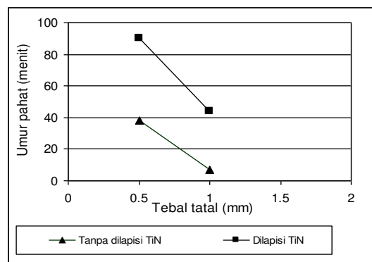
Gambar 7. Grafik tebal tatal vs umur pahat, dilapisi dan tanpa dilapisi TiN kecepatan potong 48 m/min, laju pemakanan 0.112 mm/put
