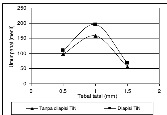
Gambar 4. Grafik tebal tatal vs umur pahat, dilapisi dan tanpa dilapisi kecepatan potong 28 m/min, laju pemakanan 0.112 mm/put
