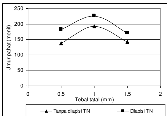
Gambar 3. Grafik tebal tatal vs umur pahat, dilapisi dan tanpa dilapisi, kecepatan potong 23 m/min, laju pemakanan 0.084 mm/put
