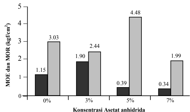
Gambar 5. MOE (■) dan MOR (□), MDF berdasarkan Konsentrasi Asetat anhidrida yang Berbeda
