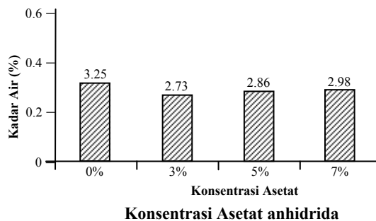
Gambar 2. Kadar Air MDF berdasarkan Konsentrasi Asetat anhidrida yang Berbeda-beda
