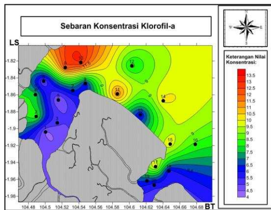
Gambar 2. Konsentrasi Klorofil-a hasil analisis laboratorium
