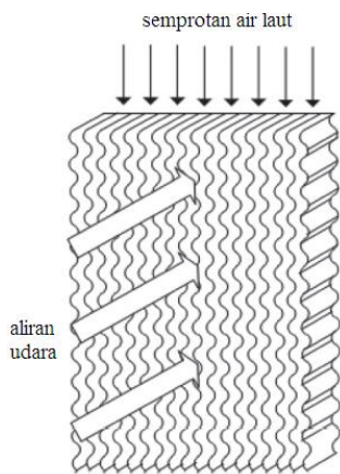
Gambar 2. Sketsa humidifier
