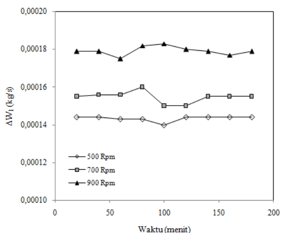
Gambar 4. Pengaruh kecepatan putaran kompresor terhadap ΔW 1
